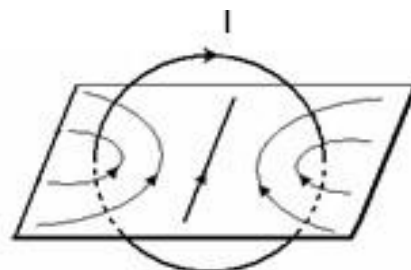
Đường sức từ của dòng điện tròn
