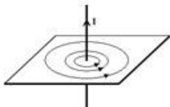
Đường sức từ của dòng điện thẳng
