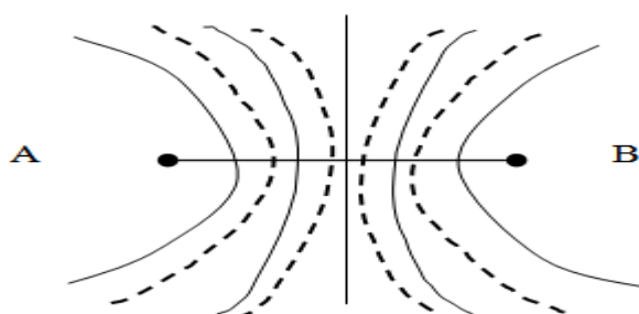
Hình 1. Giao thoa sóng âm
