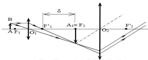
Ngắm chừng vô cực kính hiển vi
